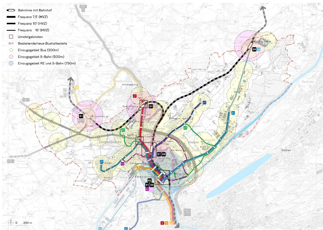
Zukünftiges Busliniennetz (Horizont 2030-35) mit Einzugsgebiet (300, 500 und 750 m)
