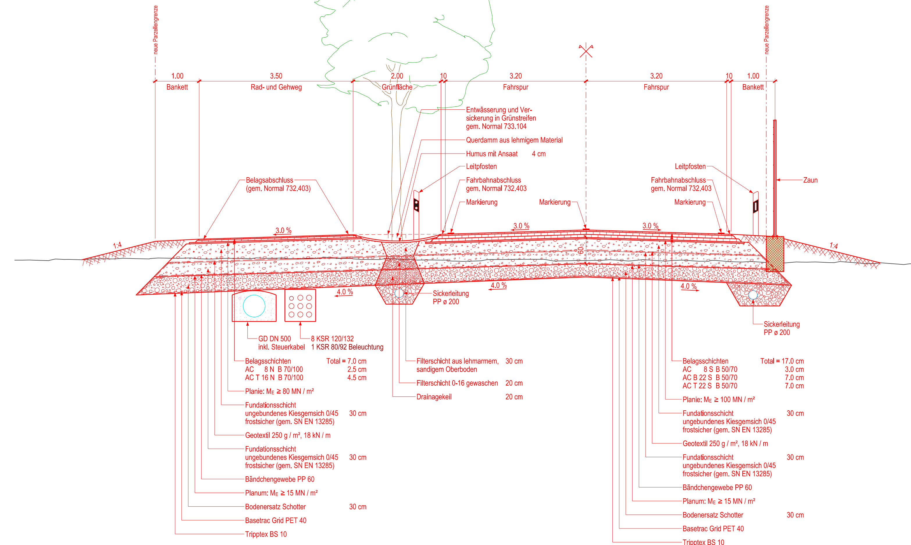
Normalprofil 1:50 m 200
