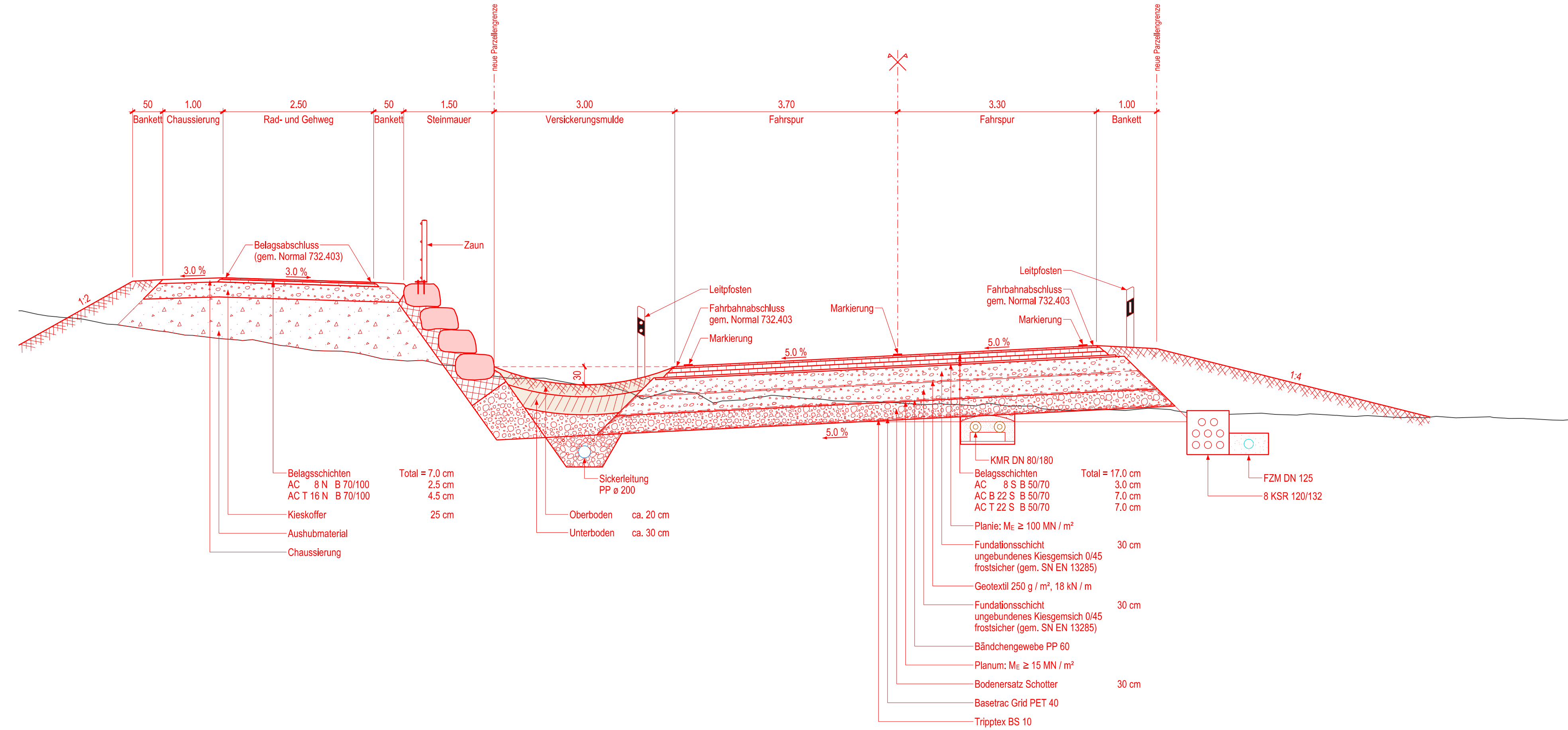
Normalprofil 1:50 m 935
