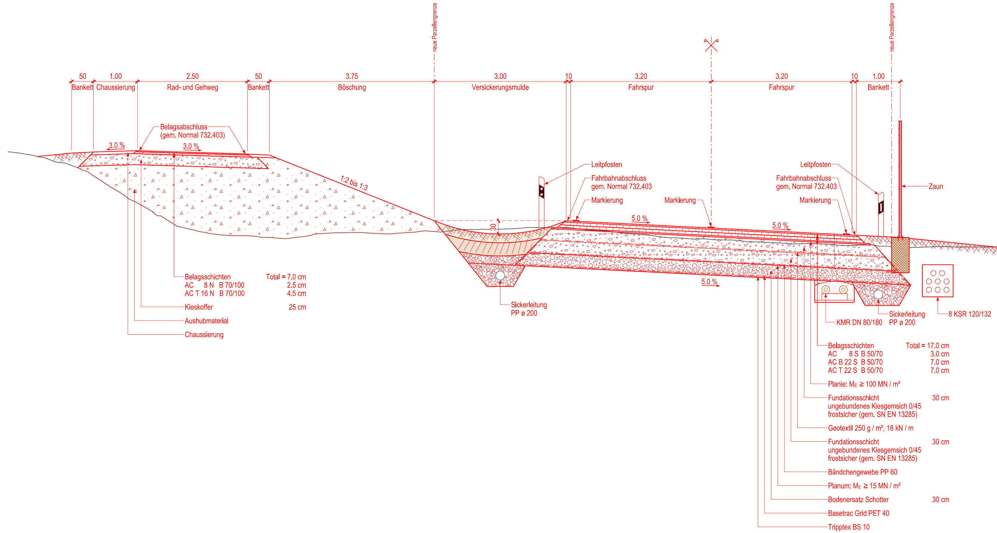
Normalprofil 1:50 m 675
