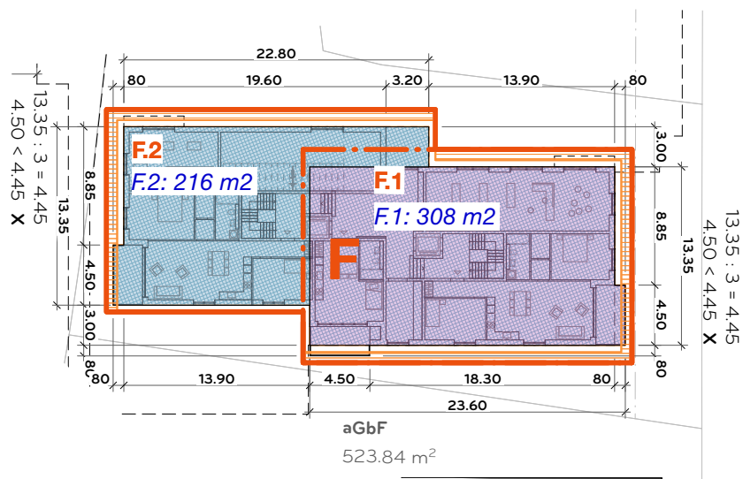
Erdgeschoss
