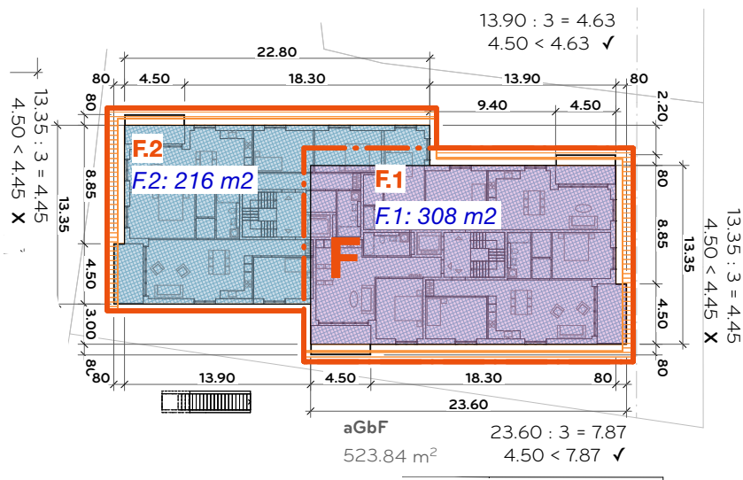
1. Obergeschoss
