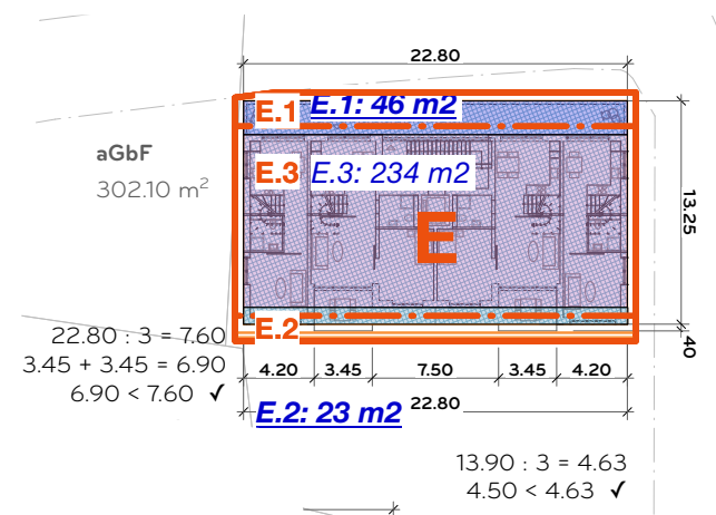
3. Obergeschoss
