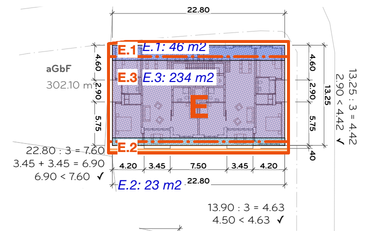
2. Obergeschoss
