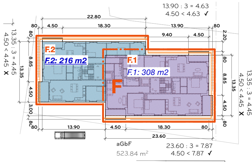
3. Obergeschoss
