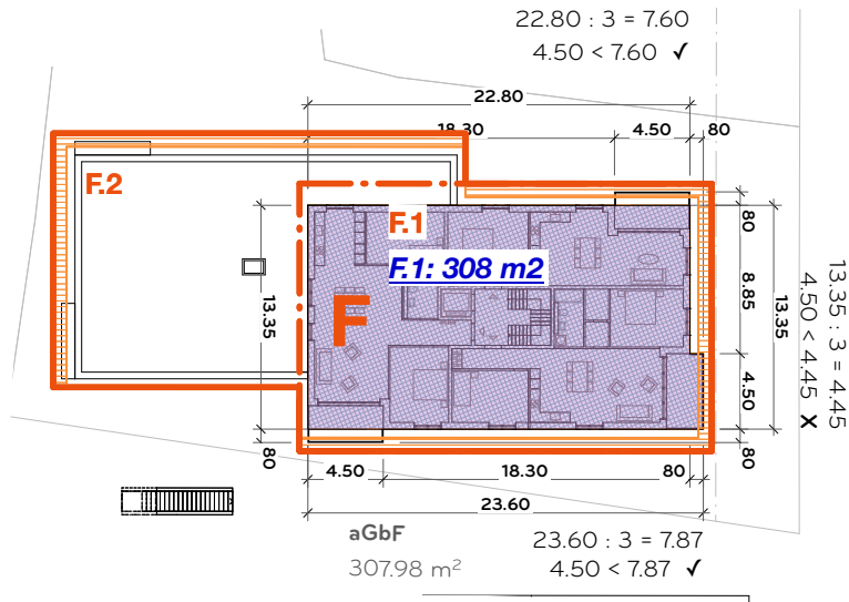
5. Obergeschoss
