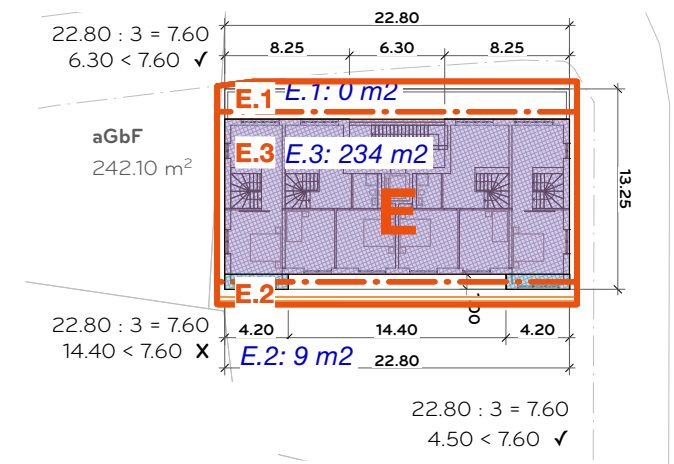
4. Obergeschoss
