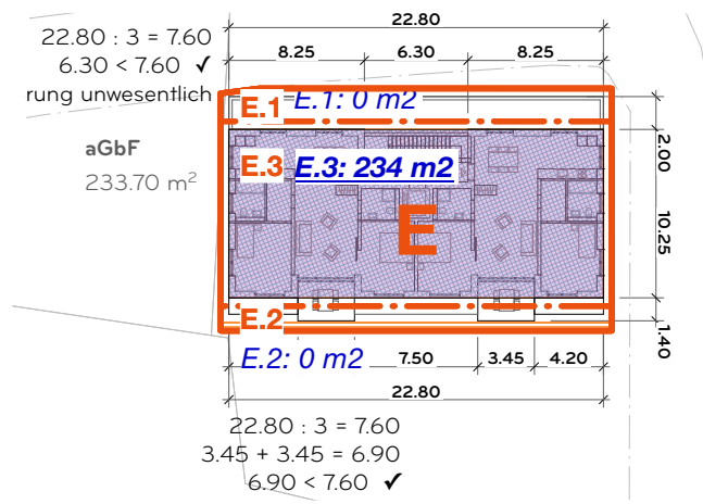
6. Obergeschoss
