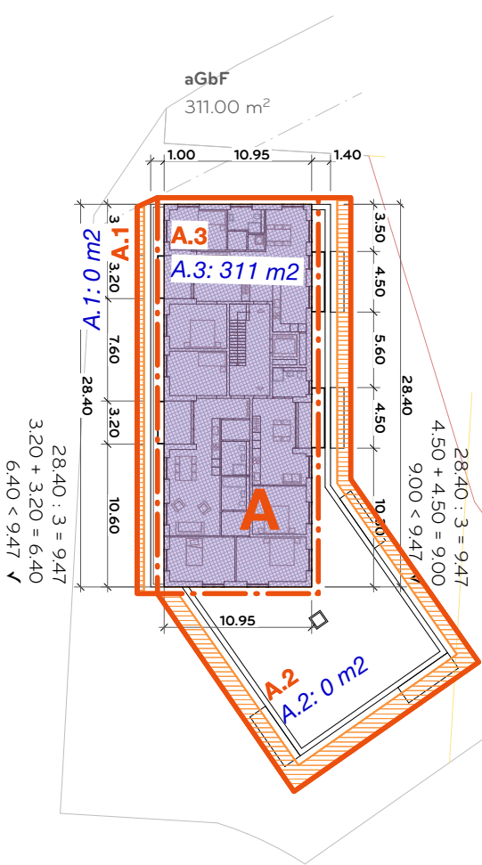
6. Obergeschoss
