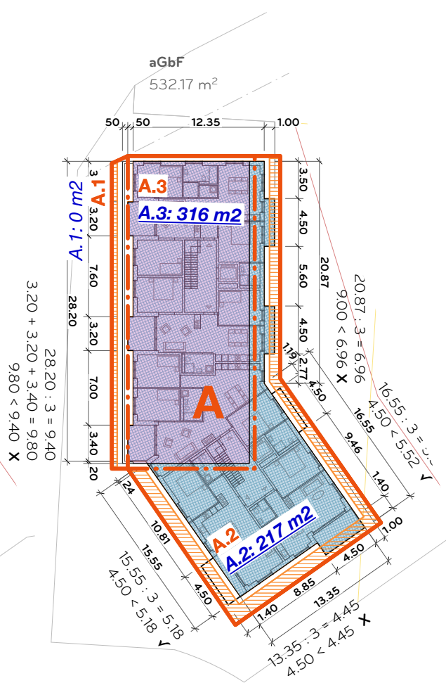
4. Obergeschoss
