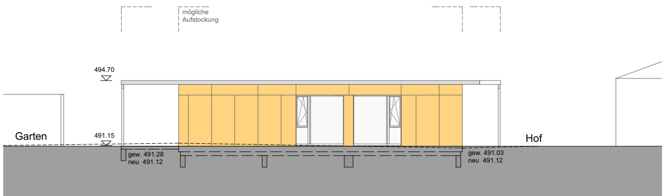
Ansicht Nord-Ost / 1:200
