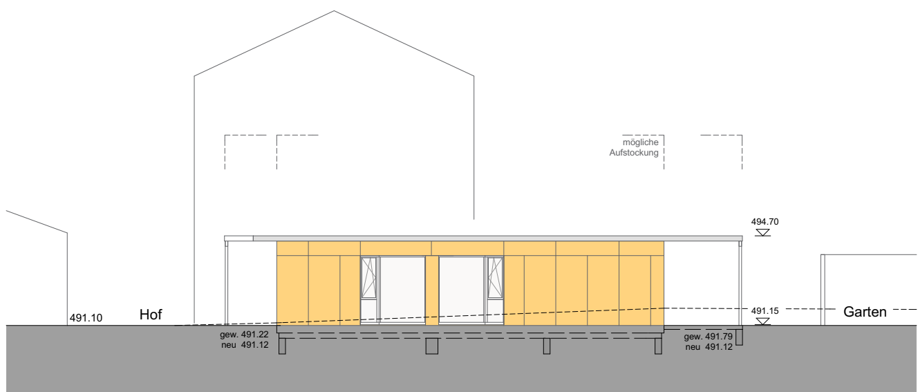
Ansicht Süd-West / 1:200
