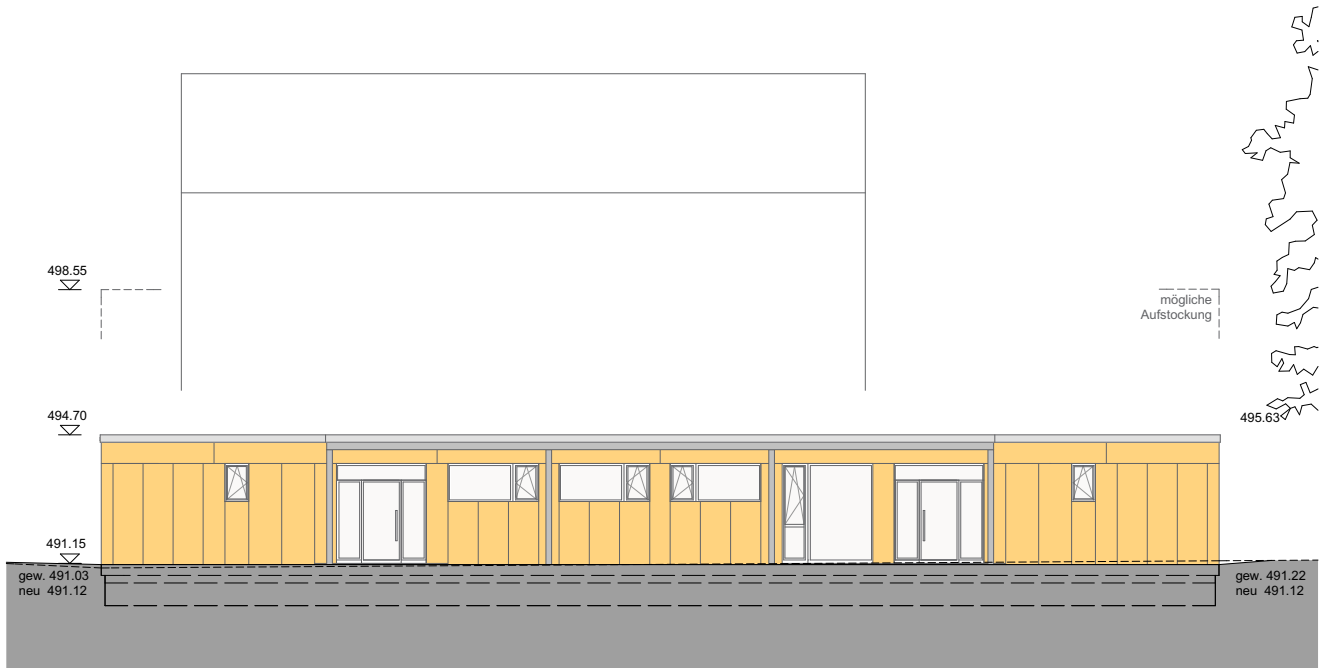
Ansicht Nord-West / 1:200
