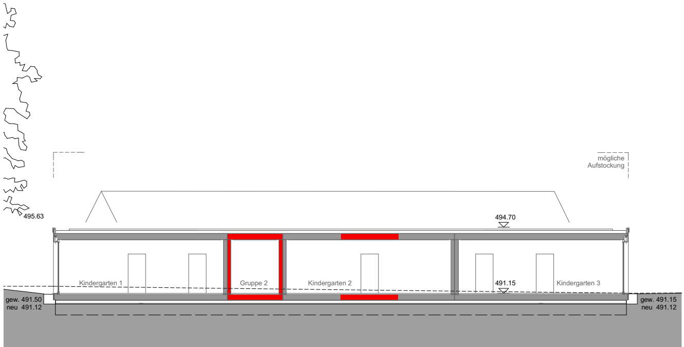
Längsschnitt / 1:200
