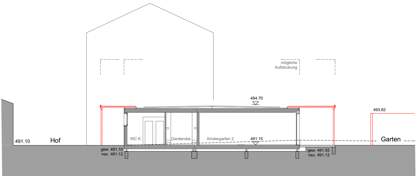
Querschnitt / 1:200
