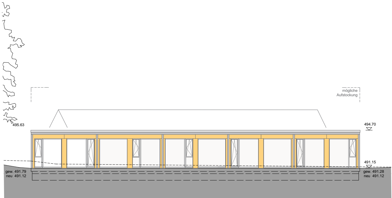
Ansicht Süd-Ost / 1:200
