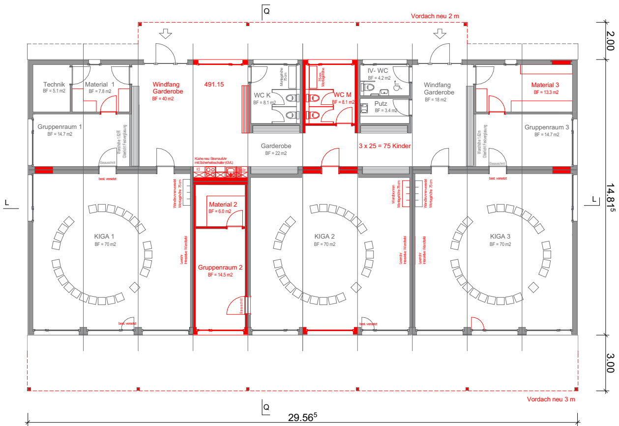
Grundriss Erdgeschoss / 1:200
